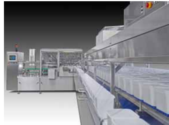
GRUNWALD-Becherfüll-Linie UF-Weißkäse
